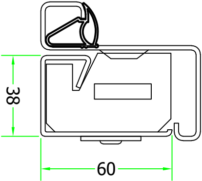
PARTICOLARE ASSEMBLAGGIO TELAIO FALSO
