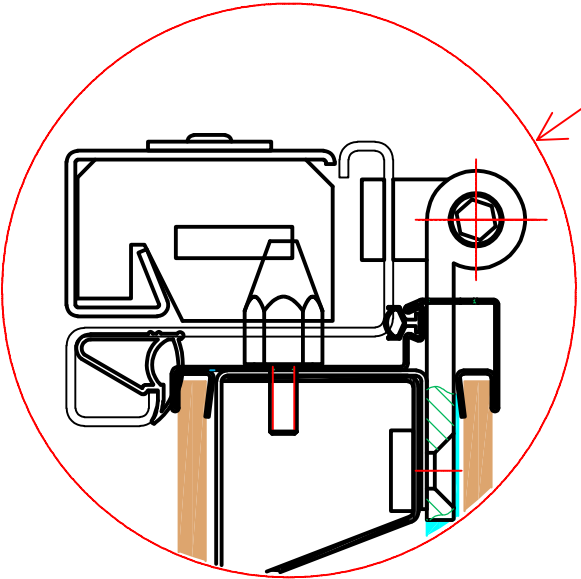
PARTICOLARE NODO LATERALE TELAIO FALSO
